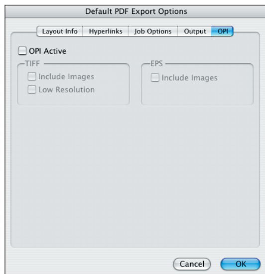
OPI
