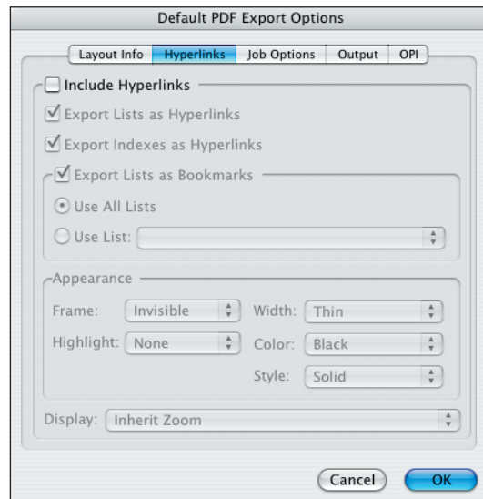
Hyperlinks
