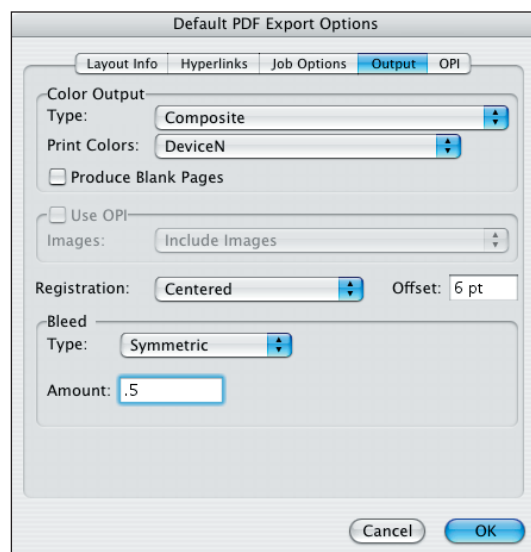
Output
